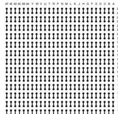
WLP676T.4C-DC260D
