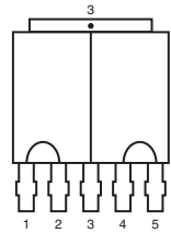
DC1245 D2PAK5
