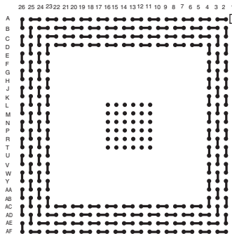
BGA388T1.27-DC72
