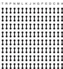
WLP256T.5C-DC168D
