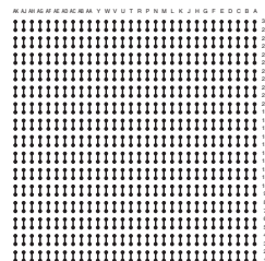
WLP900T.5C-DC307D
